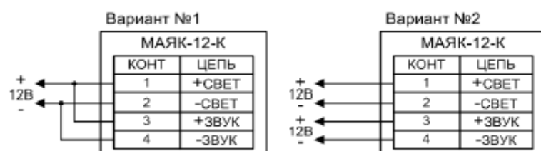
Рис.1 Схема подключения.
